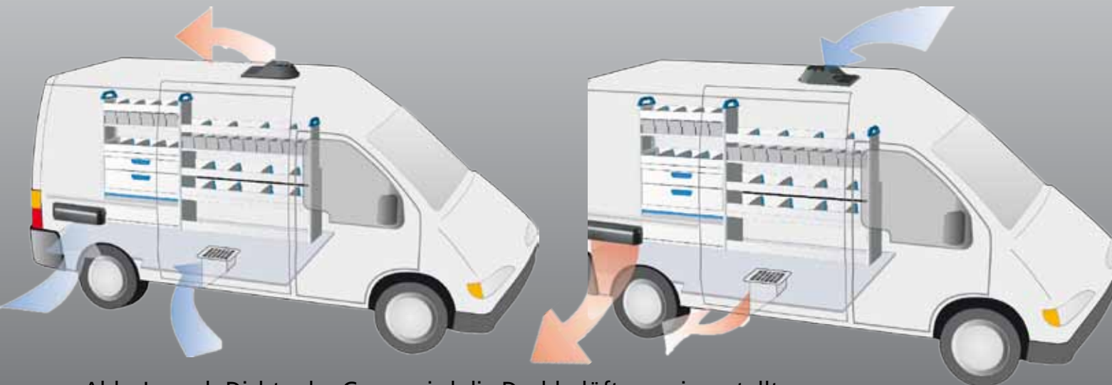
Abb: Je nach Dichte des Gases wird die Dachbelüftung eingestellt (bei großer Dichte Zuluft von oben, Entlüftung unten. bei geringer Dichte Zuluft von unten, Entlüftung oben).
